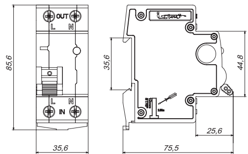
Рис. 3. Размеры УЗДП
